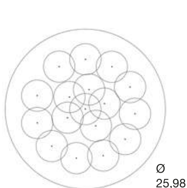
1 ZENTRALE PROBE 5 PROBEN IM 1° RADIUS 11 PROBEN IM 2° RADIUS
